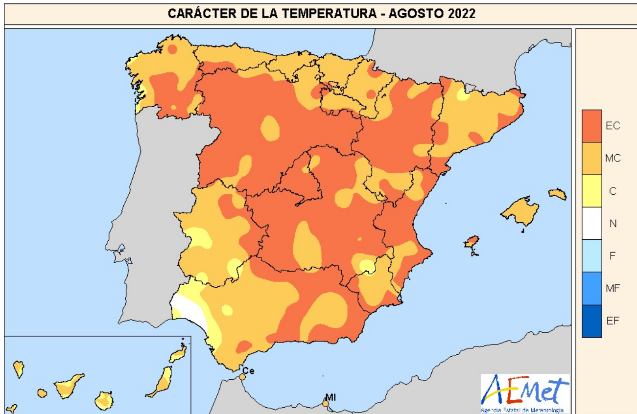
Fig. 21. Carácter de la temperatura en agosto de 2022. Fuente: AEMET
