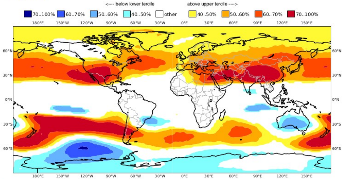
Fig. 23 Predicciones probabilísticas de geopotencial en 500 hpa. Fuente: COPERNICUS
