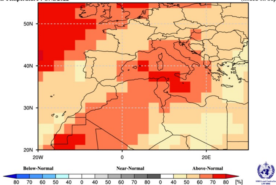
Fig 22. Predicciones probabilistas de anomalías de temperatura Fuente: https://www.wmolc.org
