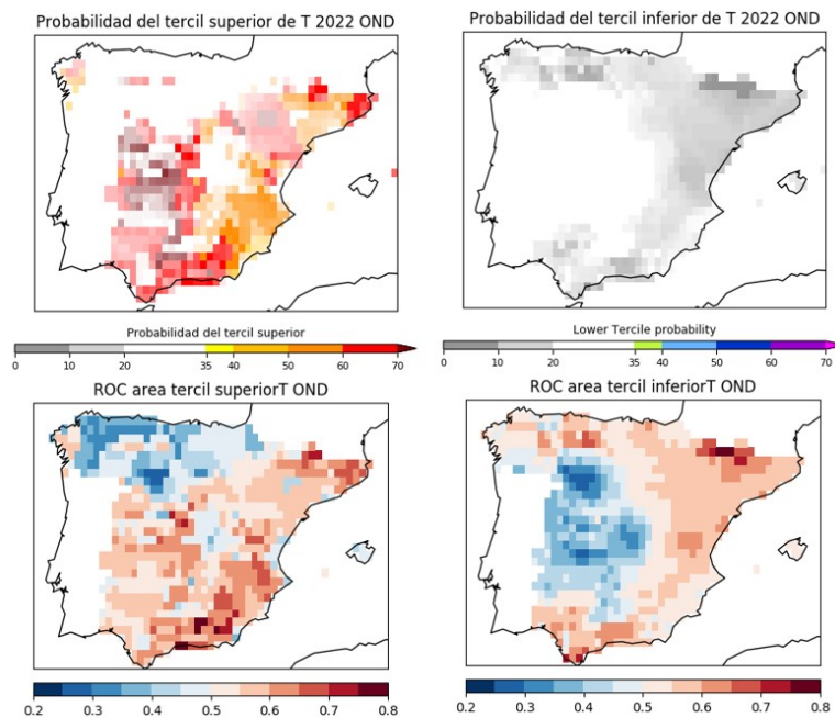
Fig.30. Predicción probabilista de temperatura ERA 5.
