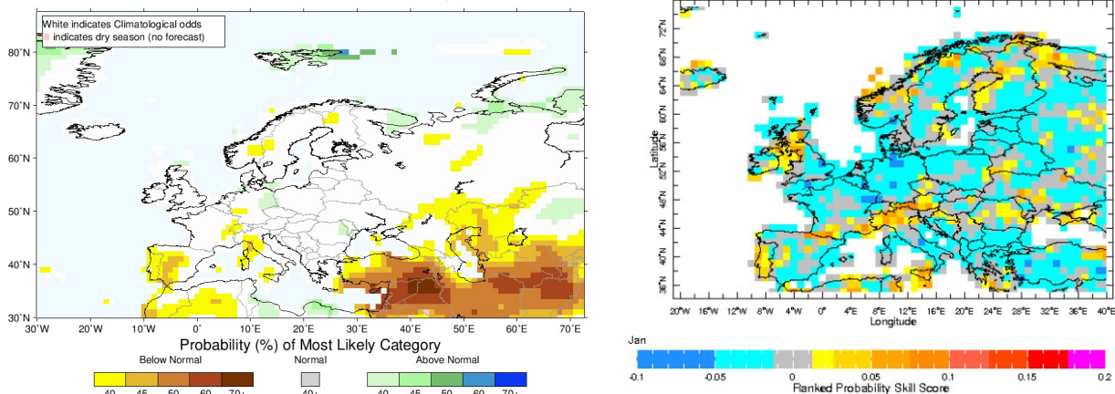
Fig. 34. Predicción probabilística y skill de anomalías de precipitación. Fuente: IRI
