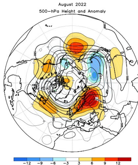
Fig. 9. Altitud y anomalías de geopotencial en agosto de 2022 en 500 hPa. Fuente: NOAA
