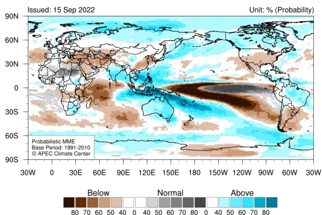
Fig. 35. Predicción probabilística de anomalías de precipitación. Fuente APCC (Apec Climate Center)
