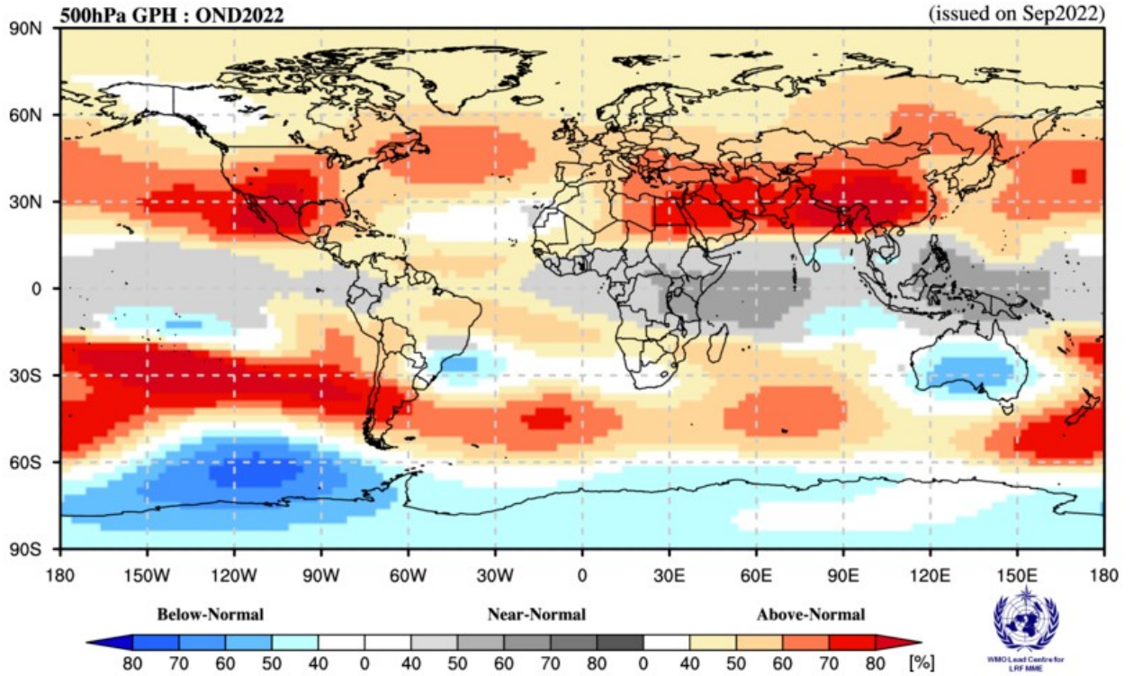
Fig 22. Predicciones probabilistas de geopotencial en 500 hpa Fuente: https://www.wmolc.org
