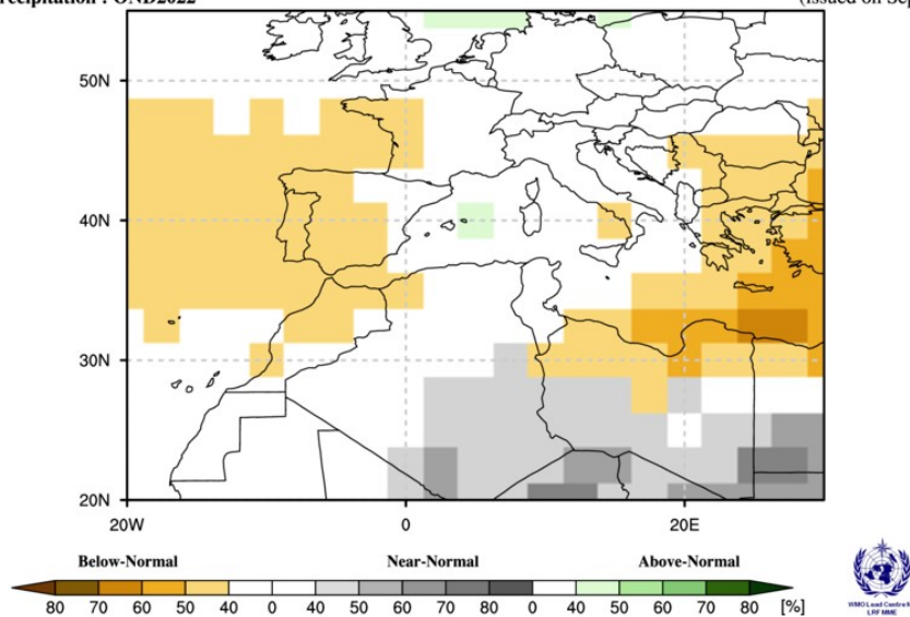
Fig 22. Predicciones probabilistas de anomalías de precipitación. Fuente: https://www.wmolc.org
