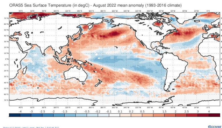
Fig. 7. Anomalía de la SST en agosto de 2022. Fuente: ECMWF
