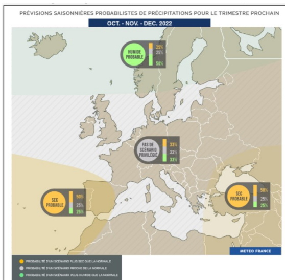
Fig 36: Predicción terciles precipitación (WMO RA VI RCC Network)
