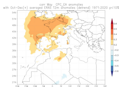
Fig.15. Correlación entre el índice EA mayo con las anomalías de temperatura a 2m en OND. Fuente https://climexp.knmi.nl
