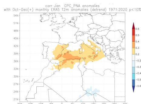
Fig.16. Correlación entre el índice PNA de enero con las anomalías de temperatura a 2m en OND. Fuente https://climexp.knmi.nl
