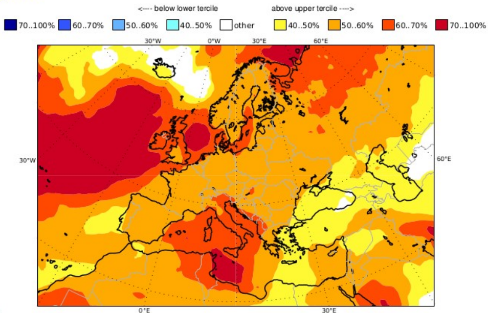
Fig. 26..Predicciones probabilísticas de temperatura a 2m. Fuente COPERNICUS
