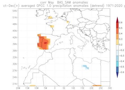
Fig.20. Correlación entre el índice SAM de mayo con las anomalías de precipitación en OND. Fuente https://climexp.knmi.nl
