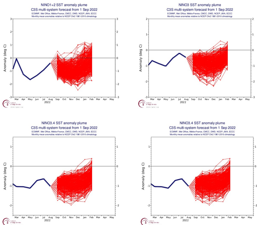
Fig. 5. Análisis y predicción del índice del Niño en las diversas regiones del Pacífico. Fuente: Copernicus
