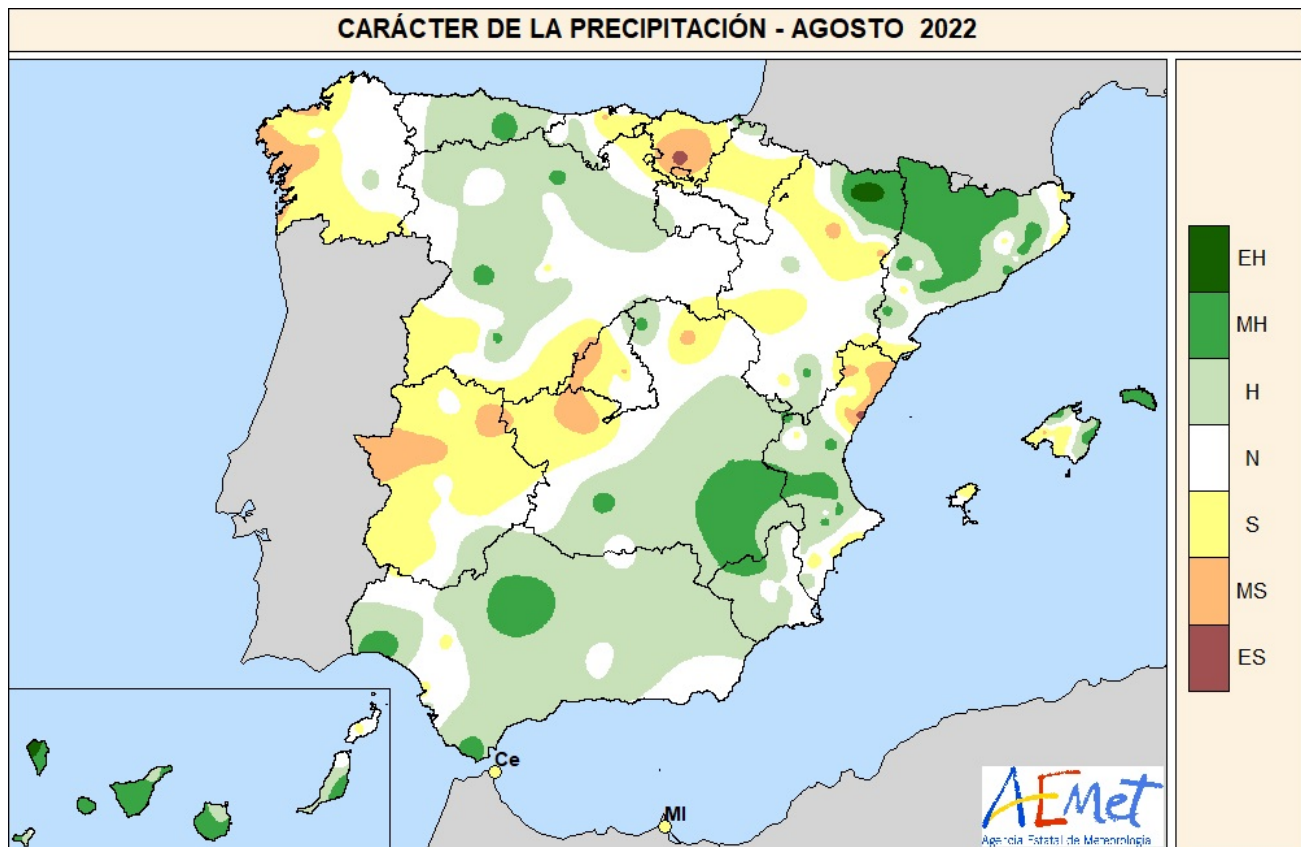
Fig. 22. Carácter de la precipitación en agosto de 2022. Fuente: AEMET
