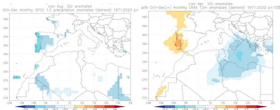
Fig.18. Correlación entre el índice SOI de agosto con las anomalías de precipitación en OND (figura izquierda) y correlación entre el índice SOI de abr con las anomalías de temperatura a 2m en OND (figura derecha) . Fuente https://climexp.knmi.nl
