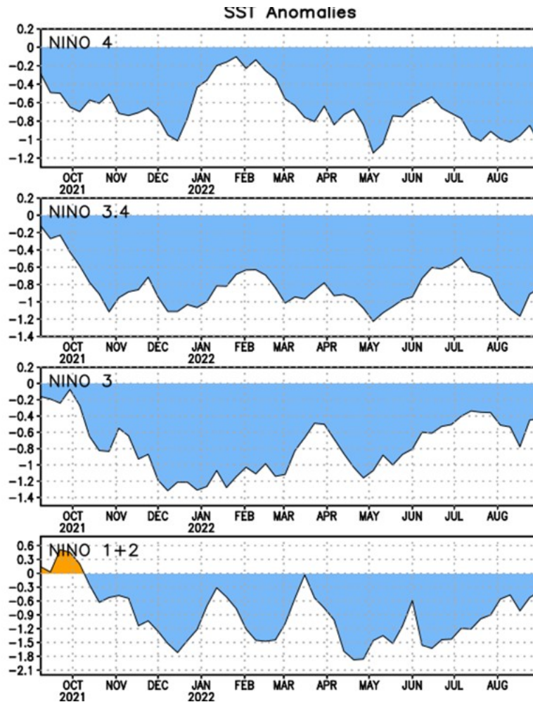
Fig. 2. Anomalías de SST en un área promediada en las regiones de El Niño. Período de referencia 1980-2010. Fuente: NOAA
