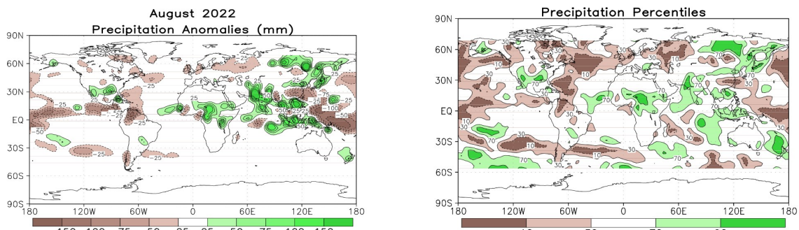
Fig. 12. Anomalía global de la precipitación en agosto de 2022 con respecto al periodo 1981-2010. Fuentes: NOAA y RCC-CM (RA-VI)
