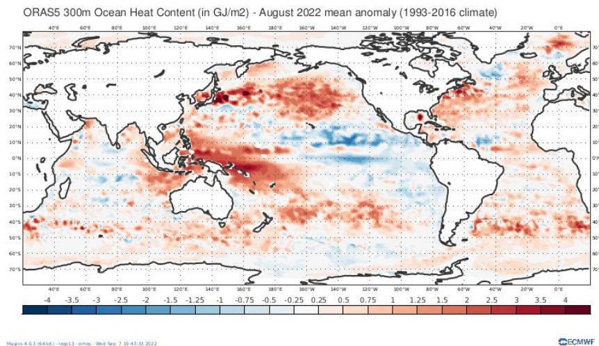
Fig. 6. Anomalía del contenido de calor acumulado en los primeros 300 m en agosto de 2022. Fuente: ECMWF
