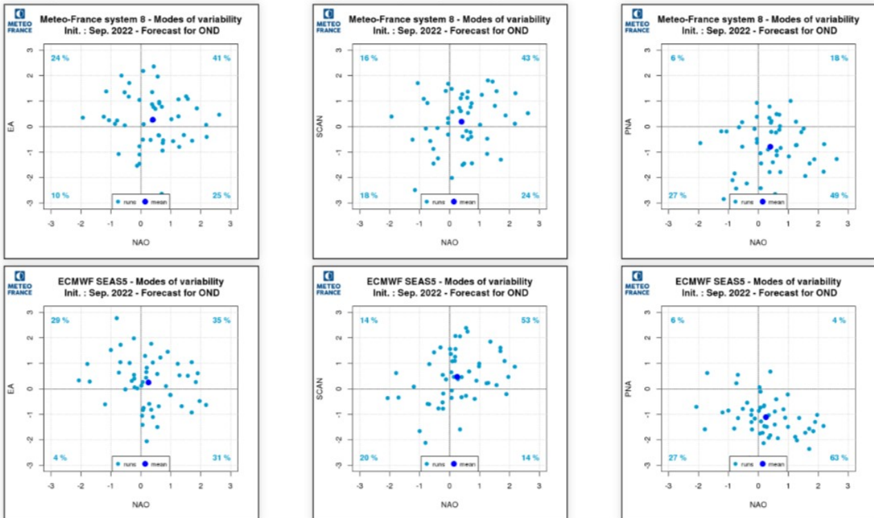
Fig. 24 Predicción modos de variabilidad. (WMO RA VI RCC Network)
