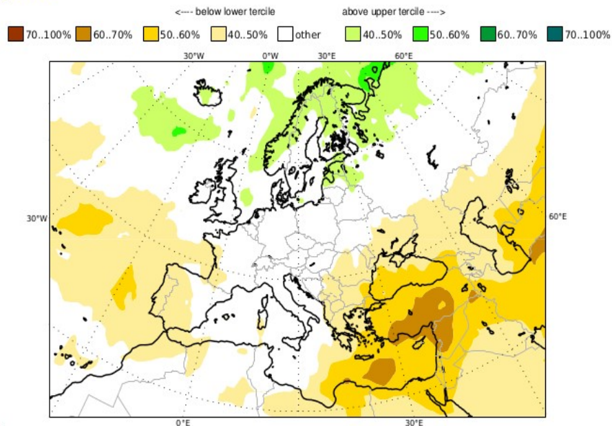
Fig. 34 Predicciones probabilísticas de precipitación. Fuente: COPERNICUS
