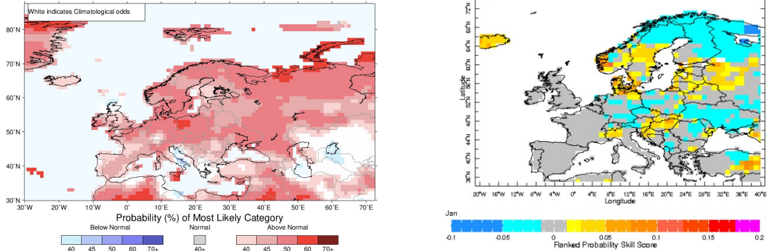
Fig. 29. Predicción probabilística y skill de terciles de temperatura. Fuente: IRI
