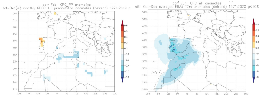
Fig.14. Correlación entre el índice WP de feb con las anomalías de precipitación en OND (figura izquierda) y correlación entre el índice WP de junio con las anomalías de temperatura a 2m en OND (figura derecha) . Fuente https://climexp.knmi.nl
