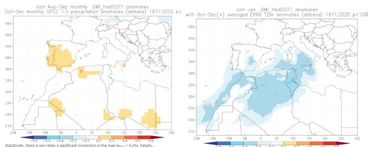
Fig.19. Correlación entre el índice DMI de ago-sep con las anomalías de precipitación en OND (figura izquierda) y correlación entre el índice DMI de enero con las anomalías de temperatura a 2m en OND (figura derecha) . Fuente https://climexp.knmi.nl
