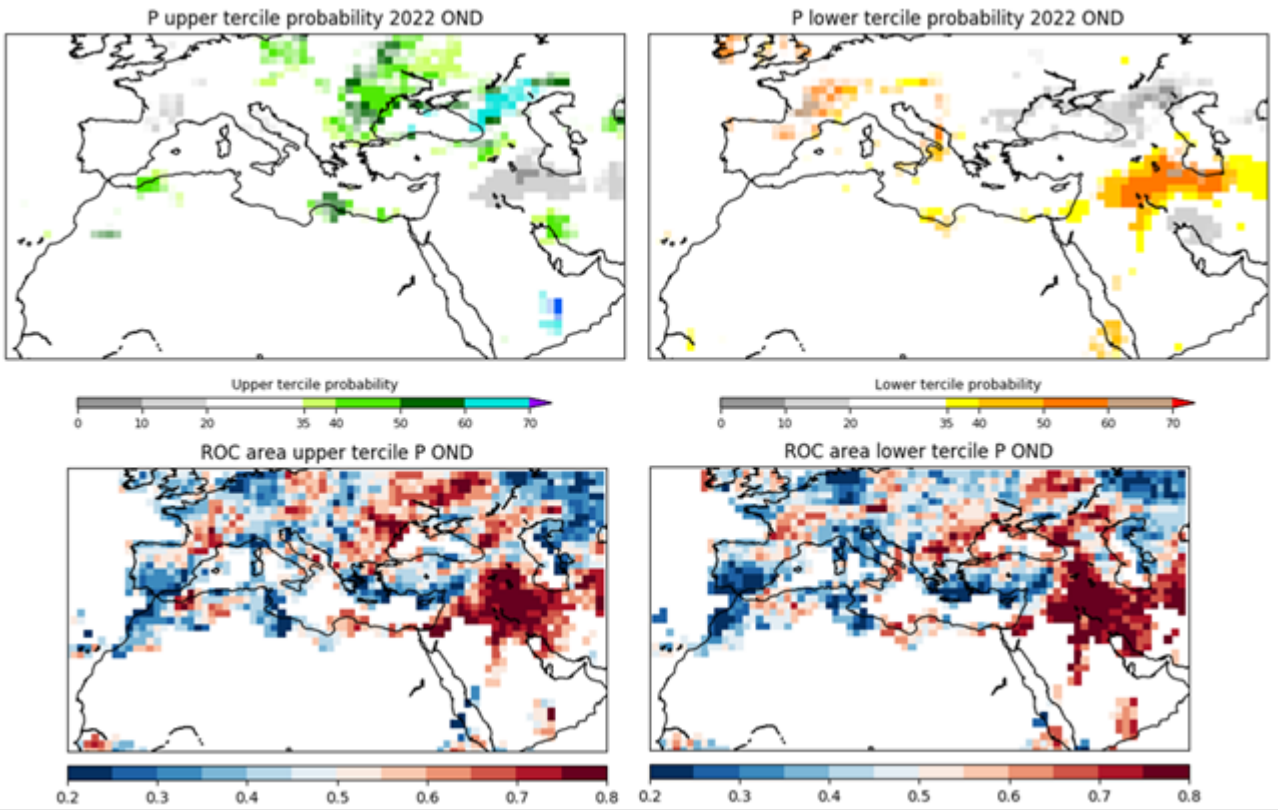
Fig.33. Predicción probabilista de anomalías de precipitación en área MEDCOF con modelo empírico AEMET.
