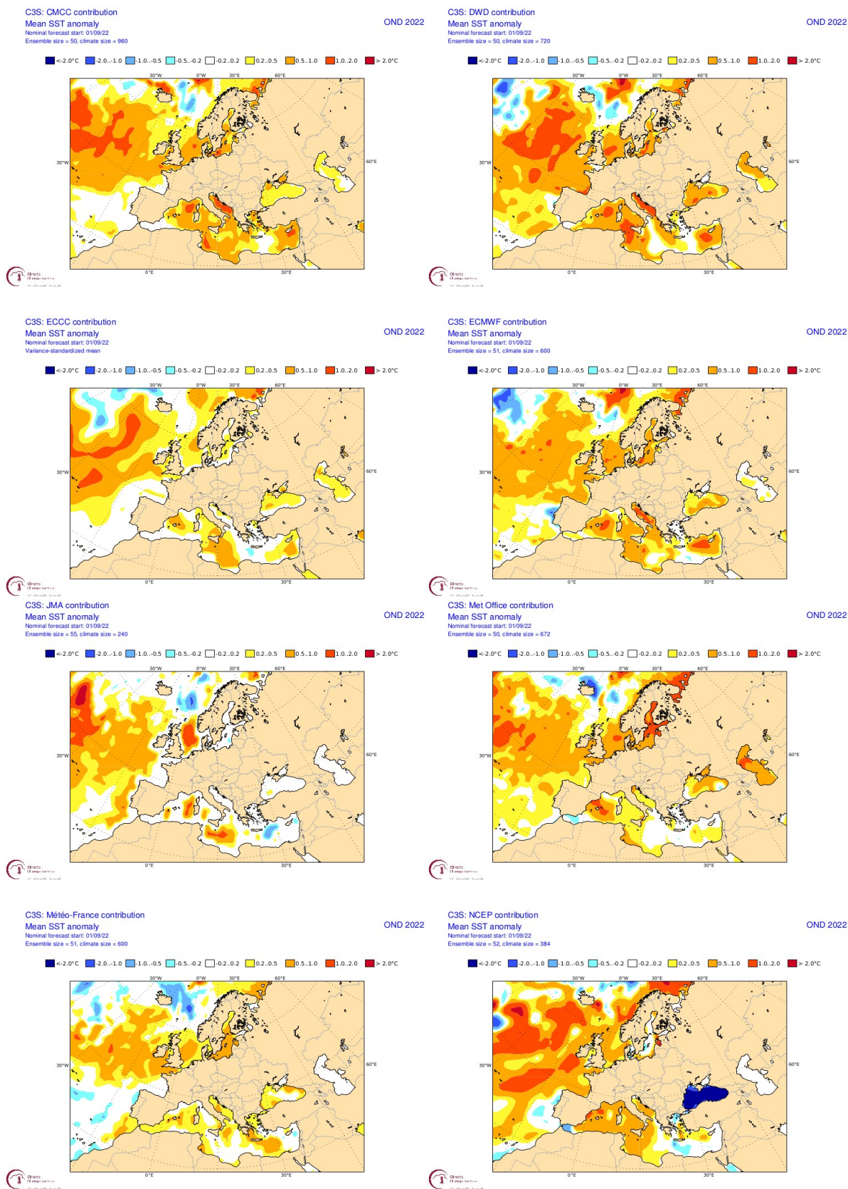
Fig. 8. Previsión de anomalía de temperatura superficial del mar para OND de 2022. Fuente: ECMWF y COPERNICUS
