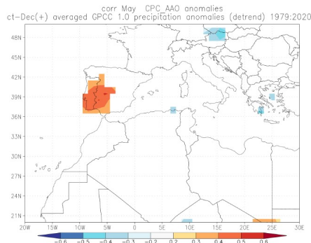
Fig.17. Correlación entre el índice AAO de mayo con las anomalías de precipitación en OND.. Fuente https://climexp.knmi.nl
