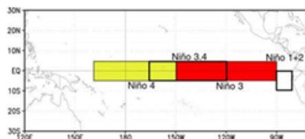
Fig. 1. Diferentes regiones Niño. Fuente:NOAA
