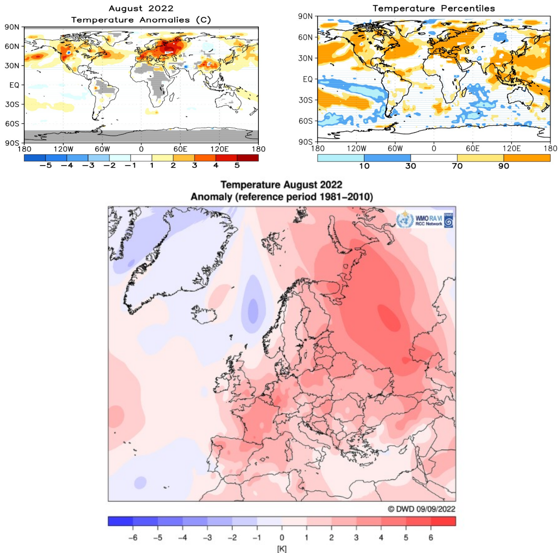
Fig. 11. Anomalía global de la temperatura en superficie en agosto de 2022 con respecto al periodo 1981-2010. Las zonas en gris indican falta de datos. Fuentes: NOAA y RCCCM
