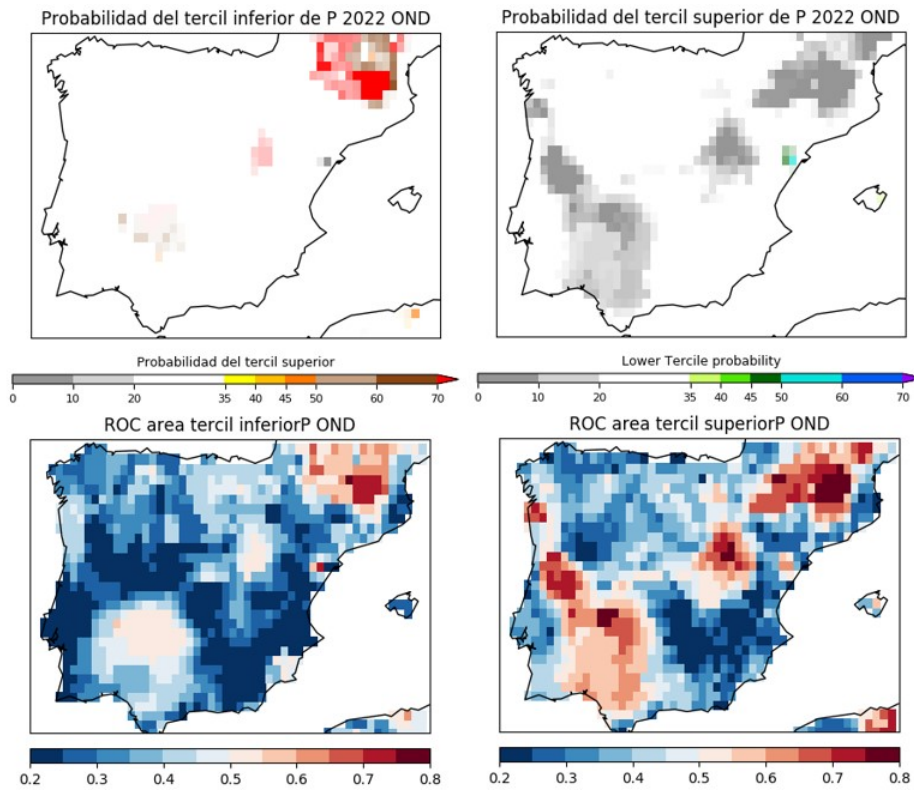
Fig.30. Predicción probabilista de precipitación EOBS.
