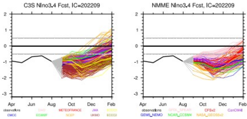
Fig. 4. Análisis y predicción del índice del Niño en la región 3.4. Fuente Medscope
